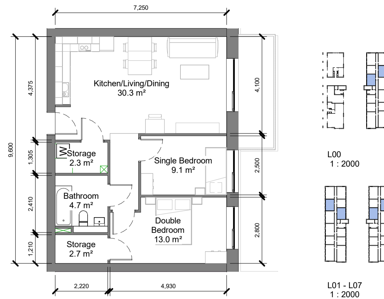
2B3P - Type 3A 1 : 100
