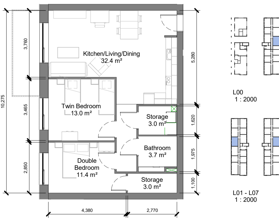
2B4P - Type 4C 1 : 100
