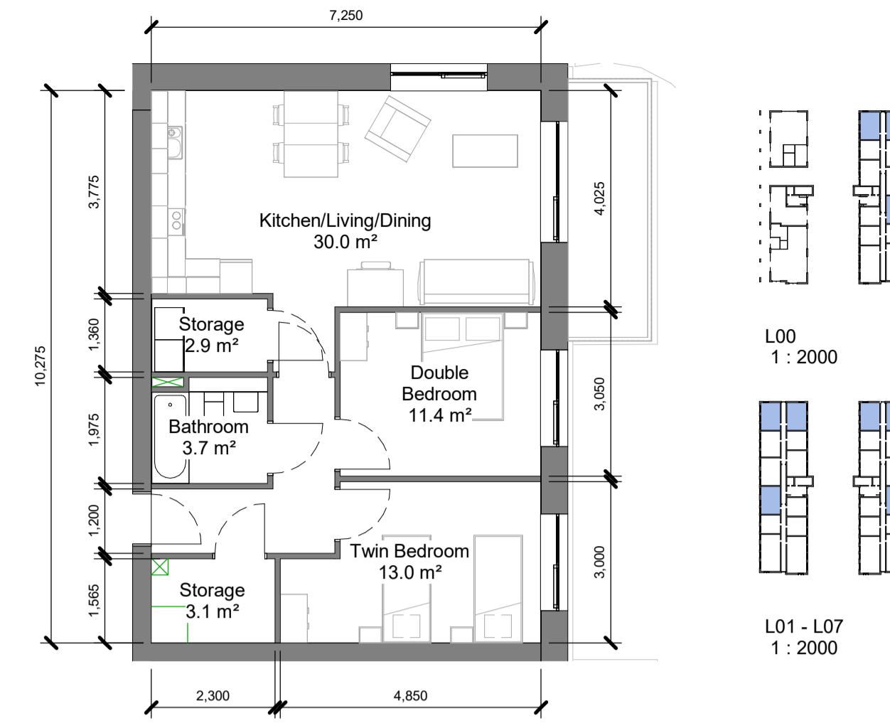
2B4P - Type 4B 1 : 100
