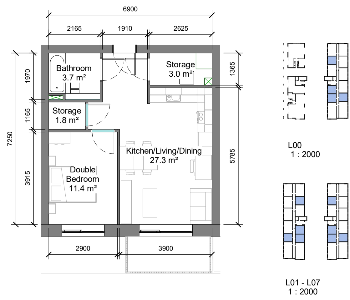
1B2P - Type 2A 1 : 100
